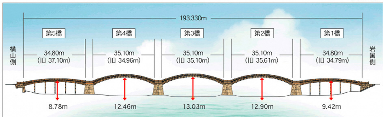
錦帯橋 側面図
