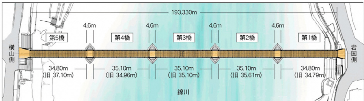
錦帯橋 平面図
