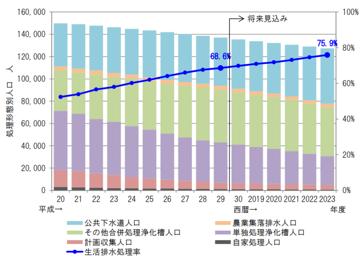
図8.30 生活排水処理の目標
