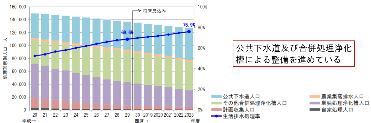
図3.5 生活排水処理の目標
