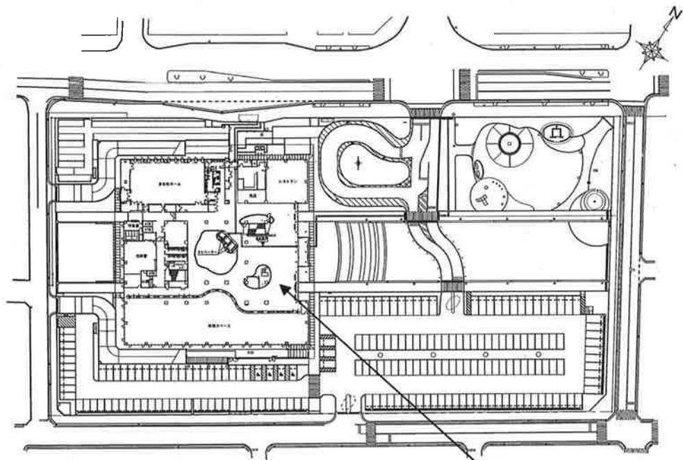
岩国市役所配置図
