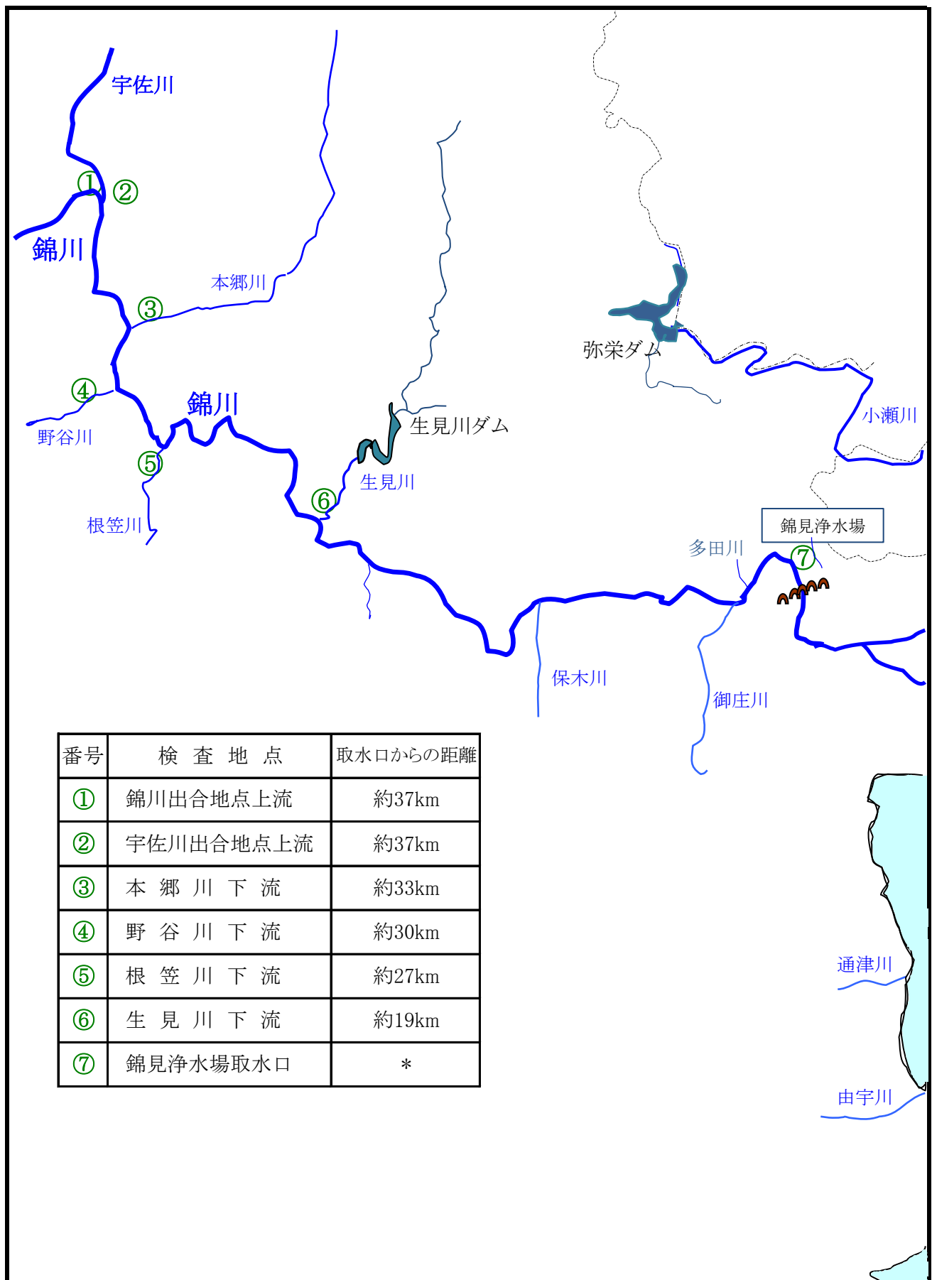
図-3 錦川水系水質調査箇所図(錦町出合地点～取水口)
