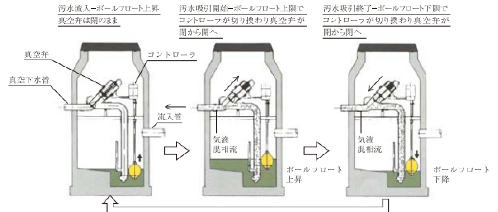
真空弁ユニットの仕組み
