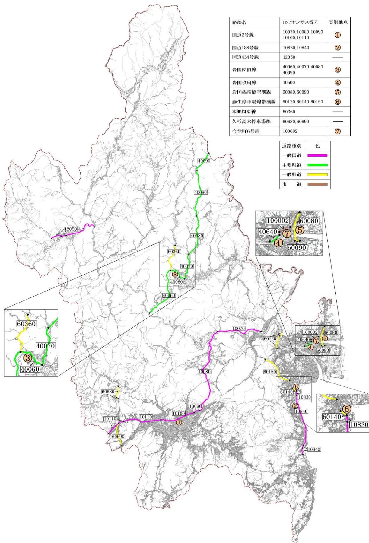
図1 自動車騒音測定地点及び面的評価路線図（平成30年度）
