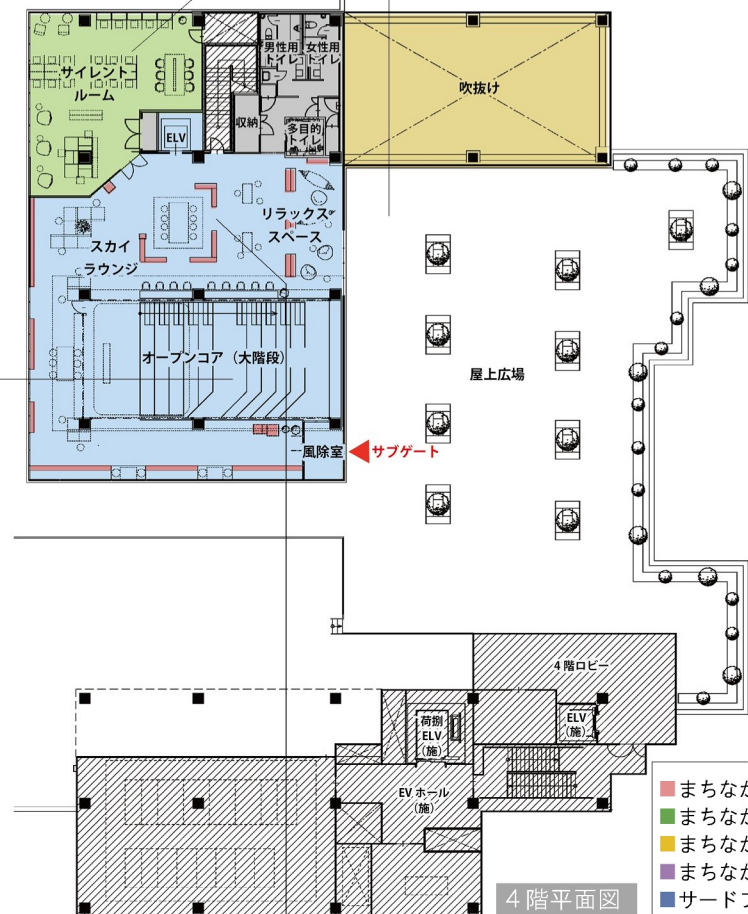
4階平面図
