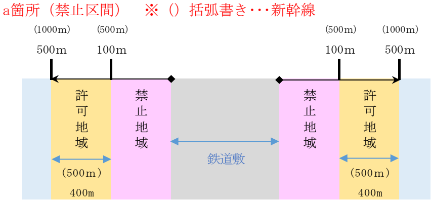
【横断図】
